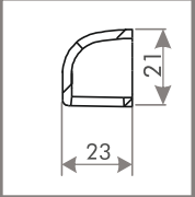
PRZEKRÓJ OZ-H 300
