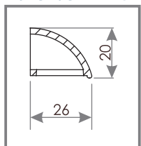
DURCHSCHNITT OZ 100
